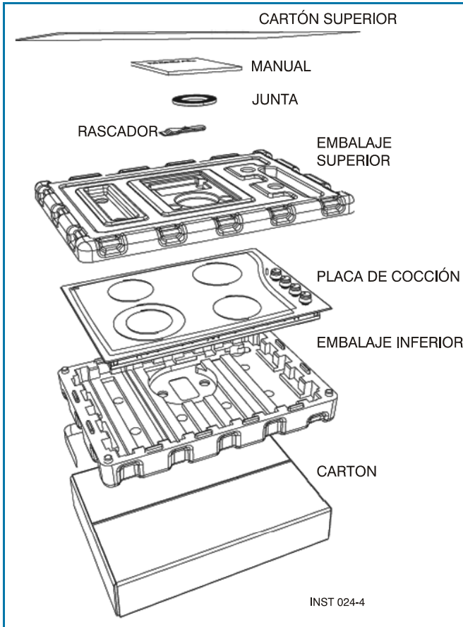
Figura 5. Piezas
